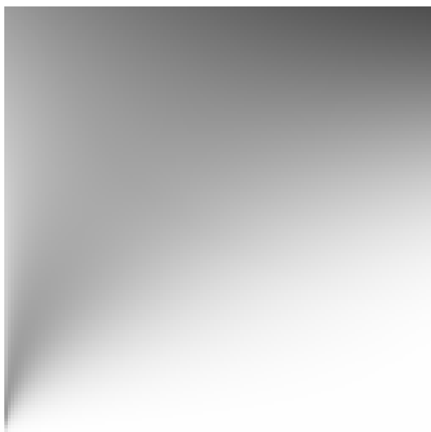
图 2: 预计算 E(\mu)
